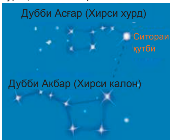
Расми 4. Бурҷи ситораҳо
