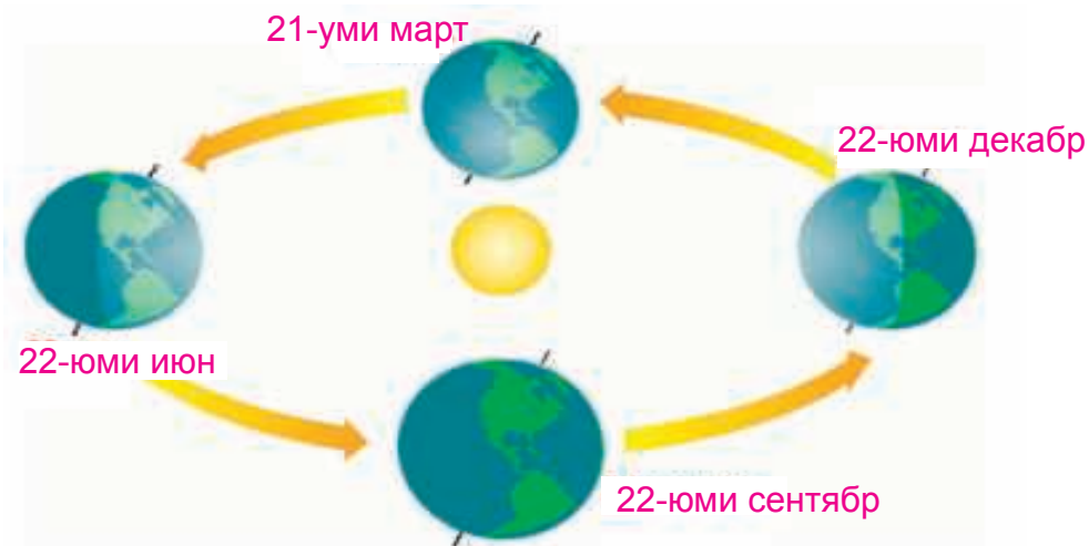
Расми 17. Ҳаракати солони Замин дар атрофи Офтоб
